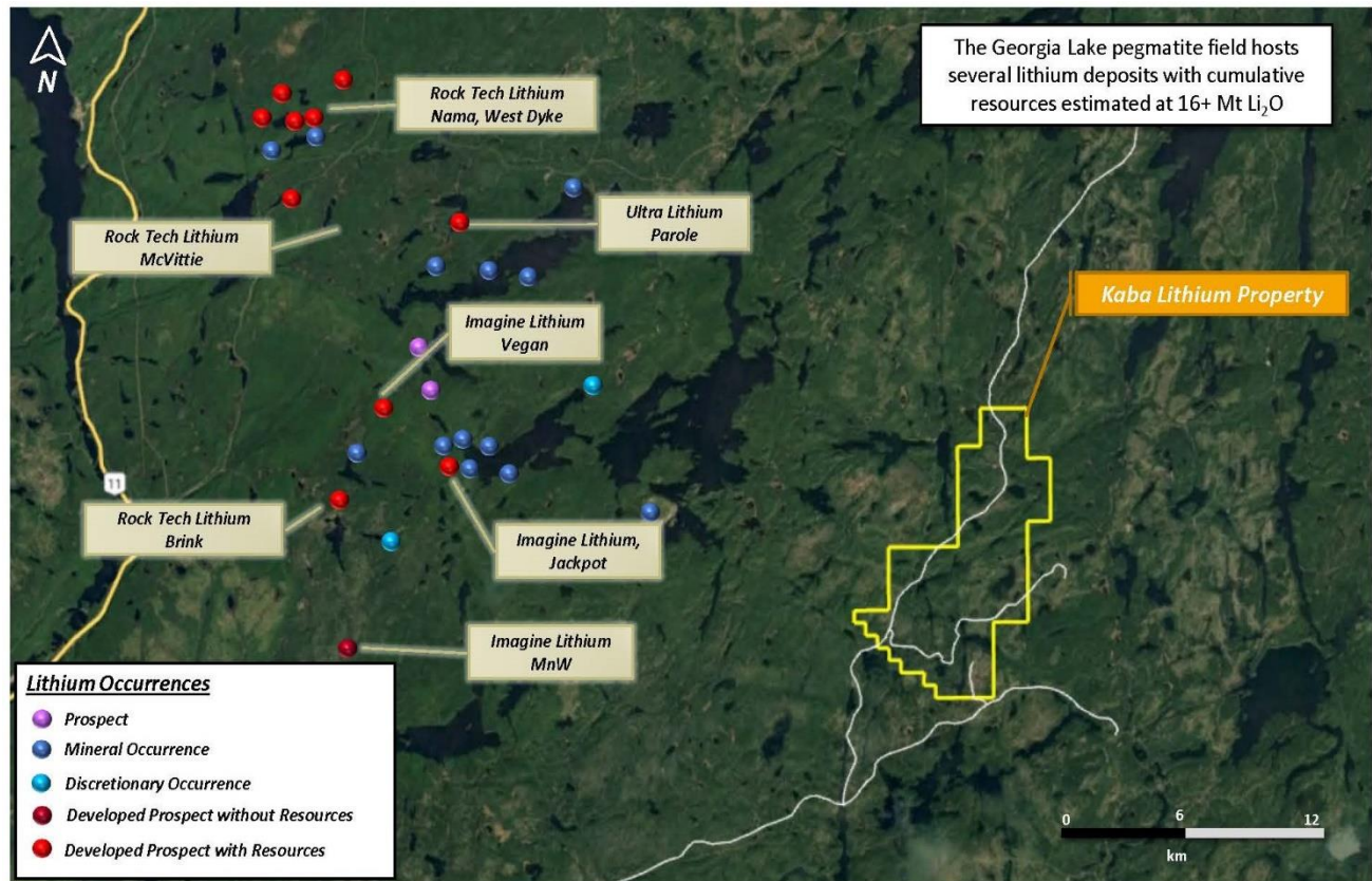
Map 1-Georgia Lake pegmatite area
