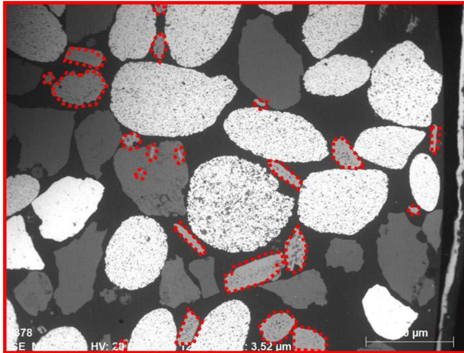
Figure 4 -Échantillon 365213 - grains analysés au MEB-EDX identifiés comme de l'ilménite (en tirt rouge).
