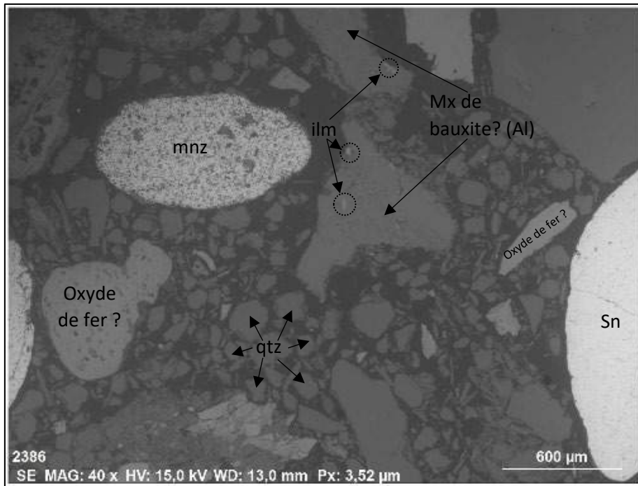
Figure 20 - Échantillon 365230 – zone analysée au MEB-EDX en identification possible des minéraux (mnz = monazite, Sn = étain, qtz = quartz, ilm = ilménite).
