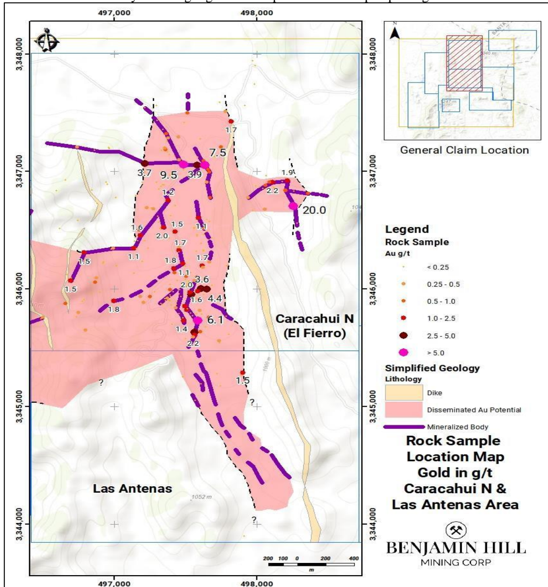
Figure. 2 - Gold assay values in g/t for the Las Antenas – Caracahui N areas (El Fierro).
