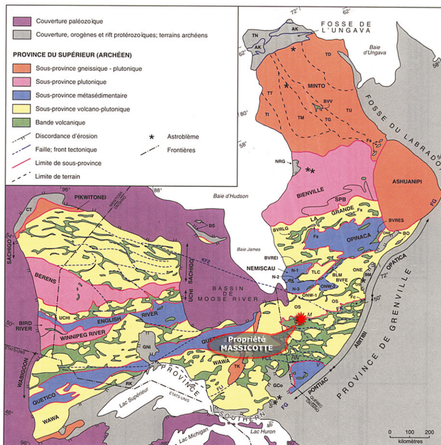
FIGURE 7: GÉOLOGIE GÉNÉRALE
