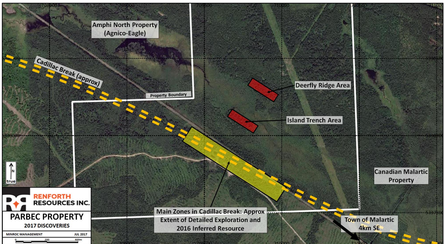
Figure 1: Carte montrant la localisation de la principale zone minéralisée au cœur de la Faille de Cadillac ainsi que les deux nouvelles découvertes dans le Groupe volcanique de Piché.
